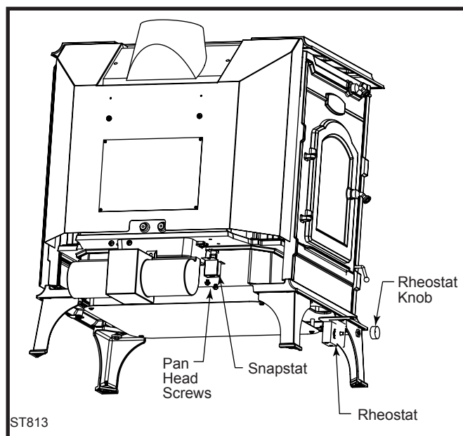
Fig. 27 Fan installation.
